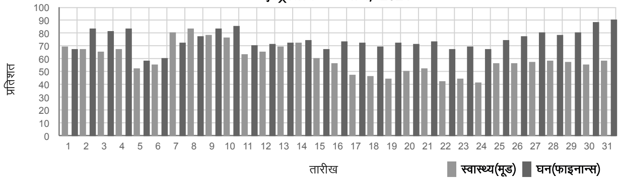
एस्ट्रोग्राफ – अप्रैल, 2024
